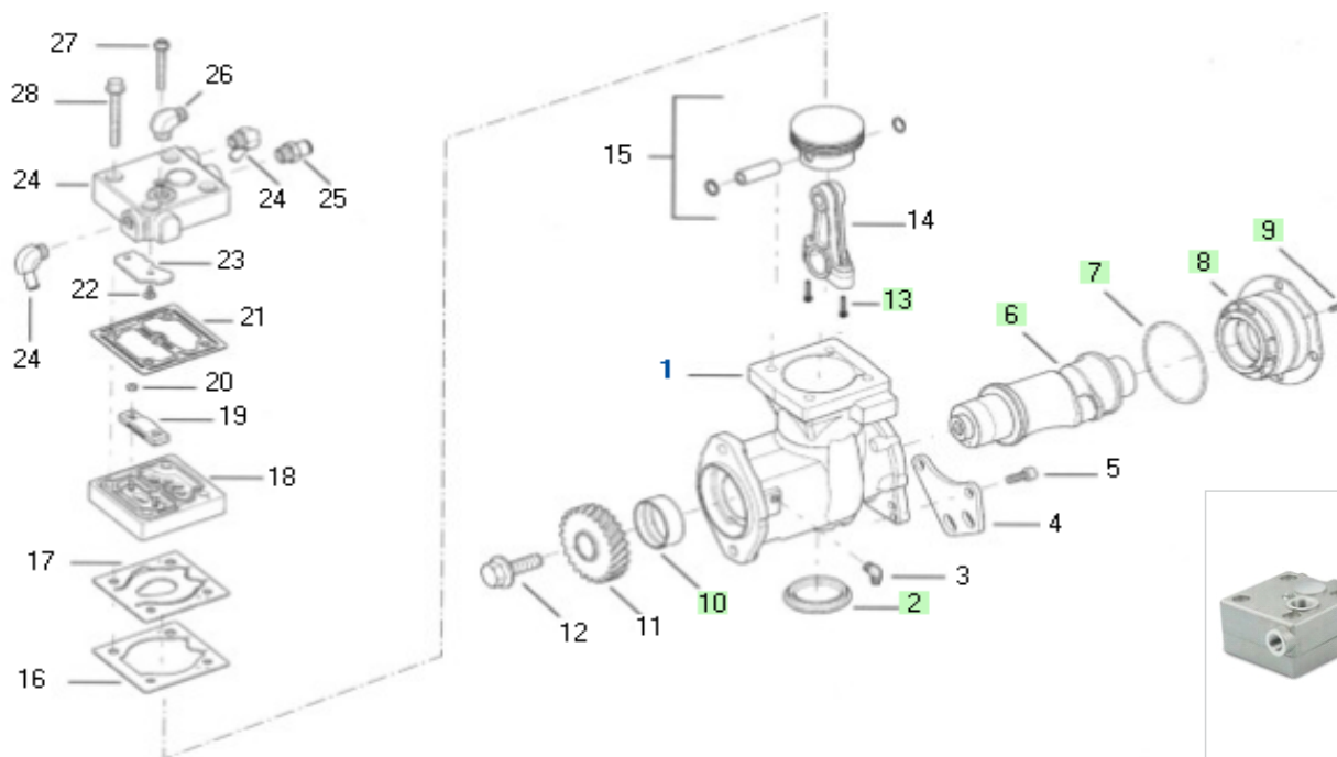
TAPA COMPLETA
